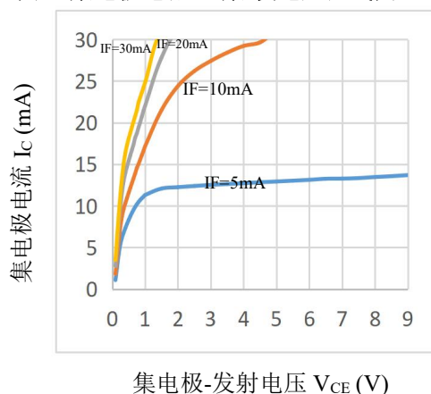
图 4. 集电极电流 vs 集-发电压曲线图
