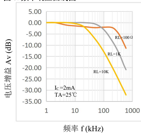
图 8. 频率响应曲线图
