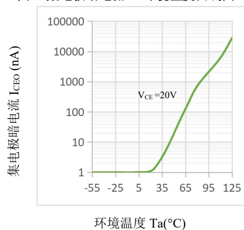
图10. 集电极暗电流 vs 环境温度曲线图
