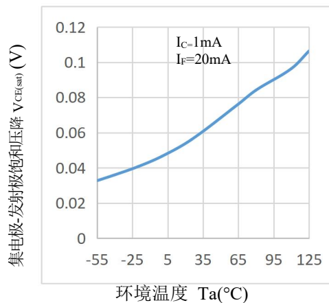
图 1. 饱和压降 vs 环境温度曲线图
