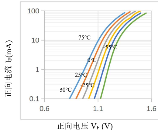
图 3. 正向电流 vs 正向电压曲线图
