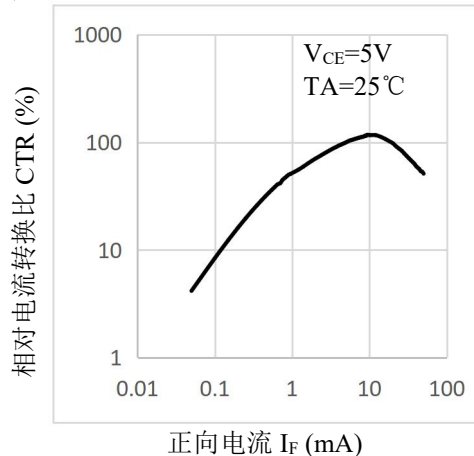
图 5. 相对电流转换比 vs 正向电流曲线图
