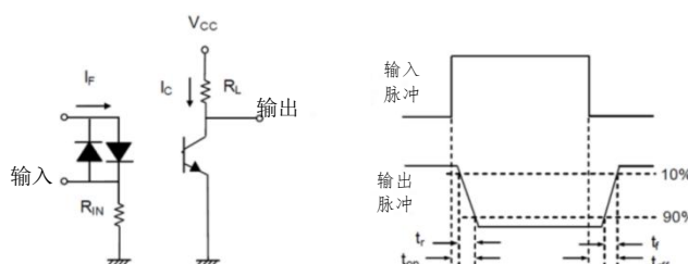
图 6. 测试线路图
