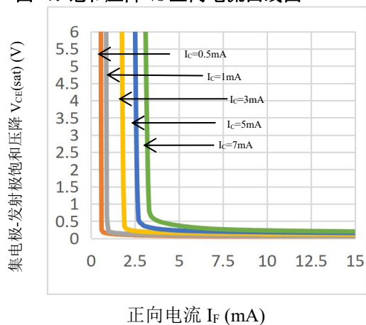
图 7. 饱和压降 vs 正向电流曲线图
