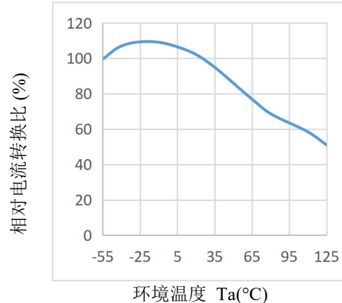
图 2. 相对电流转换比 vs 环境温度曲线图
