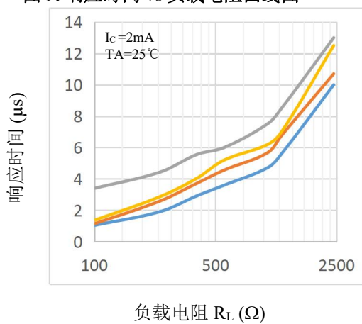
图 9. 响应时间 vs 负载电阻曲线图
